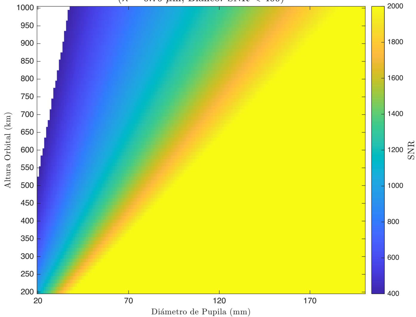
SNR - TMA - Detector 3 ( \lambda = 0.76 \mu\text{m} , Blanco: SNR < 400)
